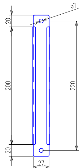
並列配管支持金具 (SD200) 平面図
