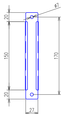
並列配管支持金具 (SD200) 平面図
