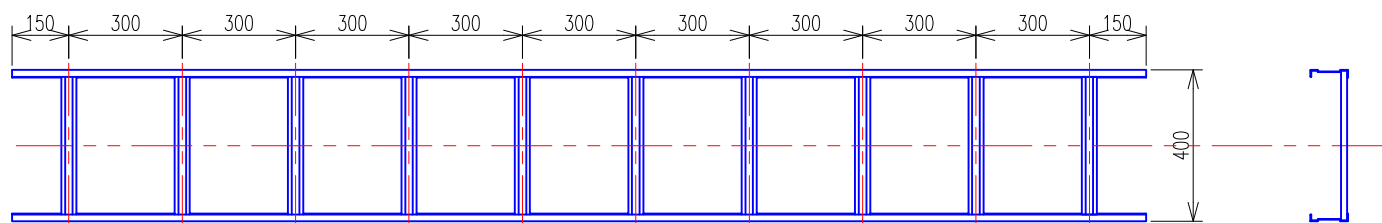
ケーブルラック (SR40) 平面図・側面図
