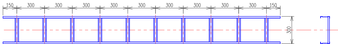
ケーブルラック (SR40) 平面図・側面図
