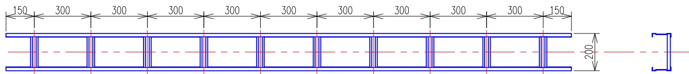
ケーブルラック (SR30) 平面図・側面図
