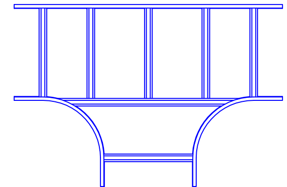
T形分岐ラック (SRT80) 平面図【ブロック】
