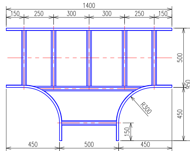
T形分岐ラック (SRT80) 平面図
