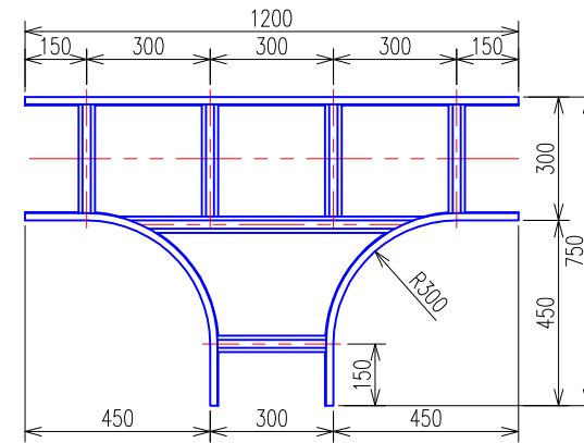
T形分岐ラック (SRT50) 平面図
