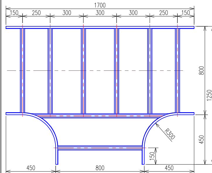
T形分岐ラック (SRT80) 平面図
