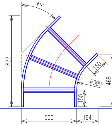
水平ベンドラック (SRA560) 平面図
