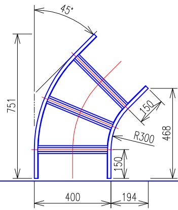
水平ベンドラック (SRA460) 平面図
