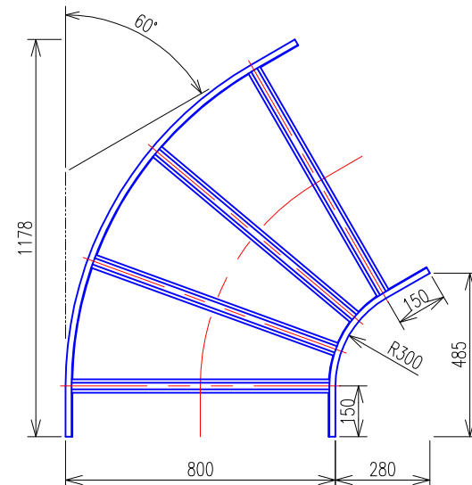
水平ベンドラック (SRA860) 平面図
