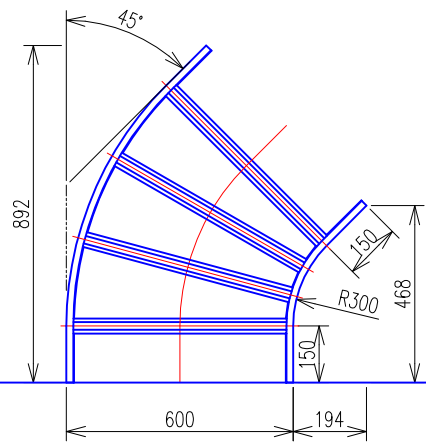
水平ベンドラック (SRA660) 平面図
