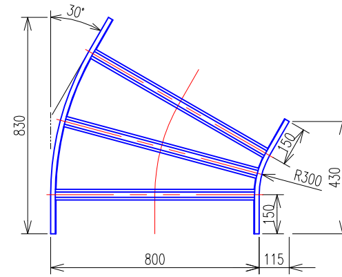
水平ベンドラック (SRA830) 平面図
