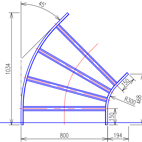
水平ベンドラック (SRA860) 平面図
