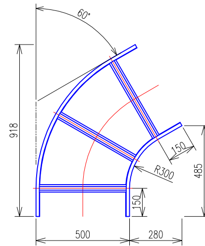
水平ベンドラック (SRA560) 平面図
