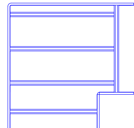
内・外直角L形分岐ラック (SRLAC80) 平面図【ブロック】
