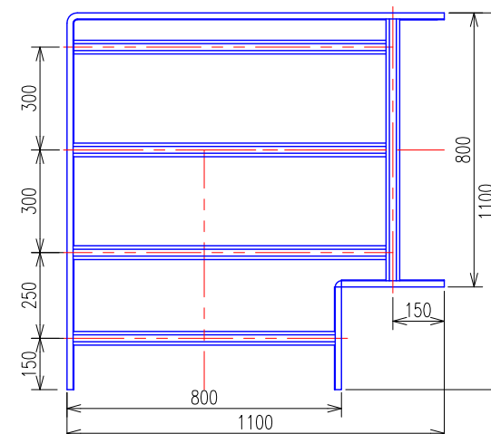
内・外直角L形分岐ラック (SRLAC80) 平面図
