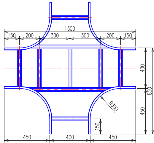
X形分岐ラック (QRX60) 平面図
