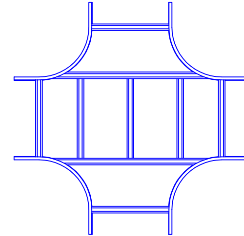
X形分岐ラック (QRX50) 平面図【ブロック】
