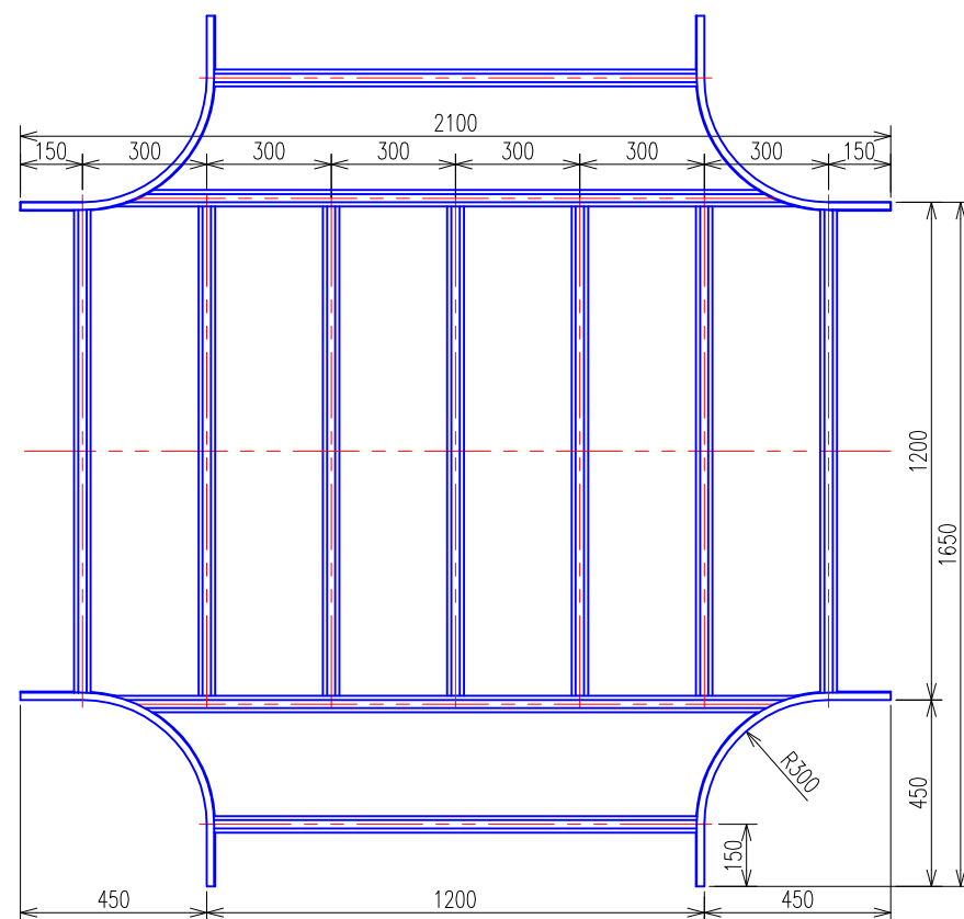
X形分岐ラック (QRX120) 平面図
