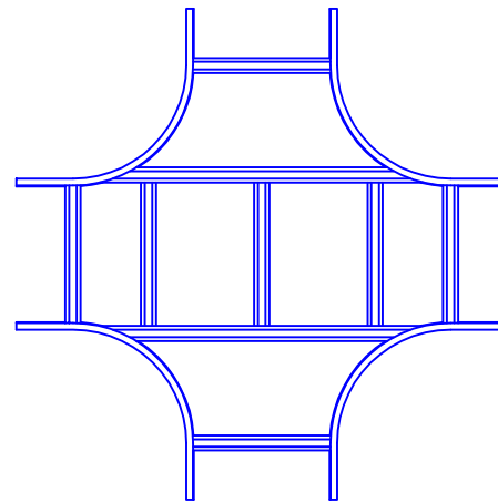
X形分岐ラック (QRX40) 平面図【ブロック】
