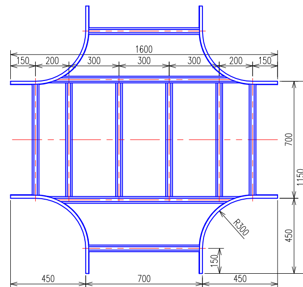
X形分岐ラック (QRX70) 平面図
