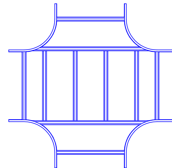
X形分岐ラック (QRX70) 平面図【ブロック】
