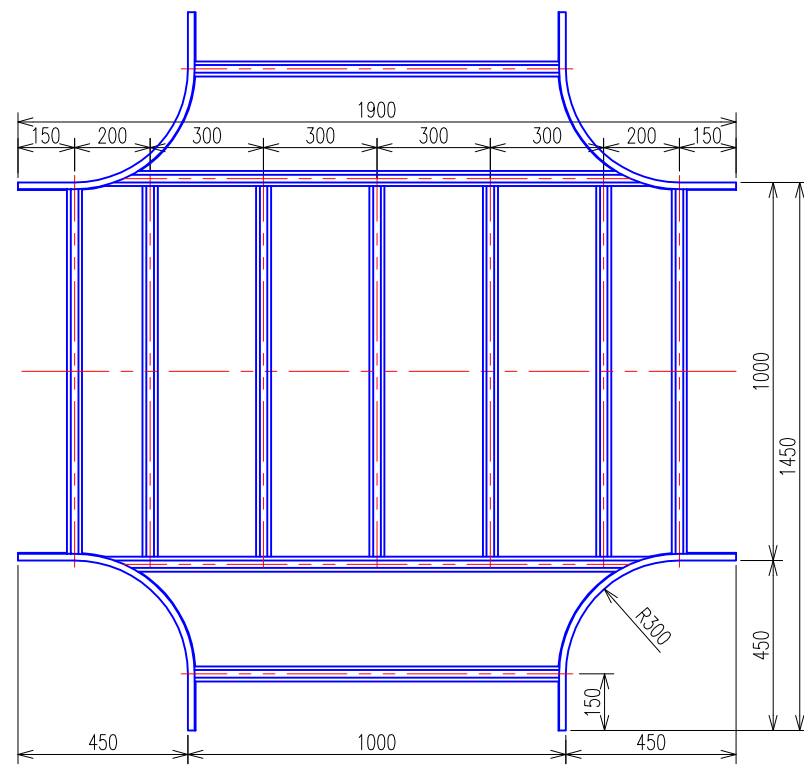
X形分岐ラック (QRX120) 平面図
