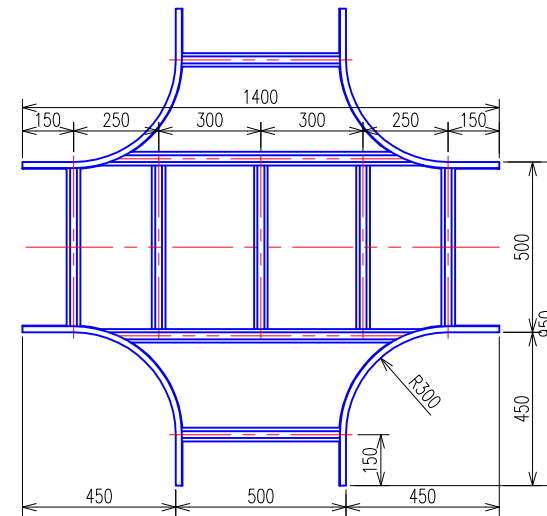
X形分岐ラック (QRX70) 平面図
