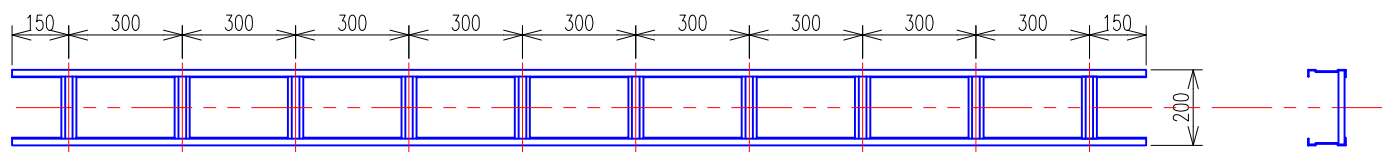
ケーブルラック (QR30) 平面図・側面図
