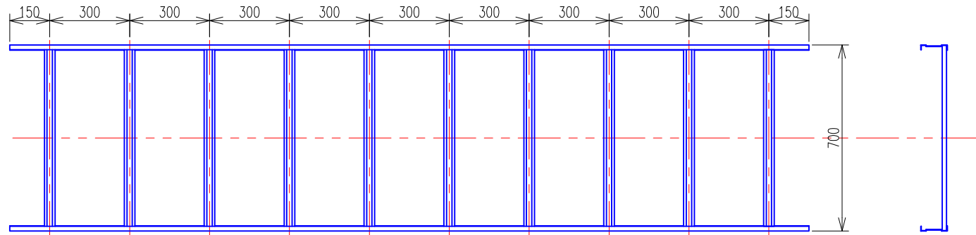
ケーブルラック (QR80) 平面図・側面図
