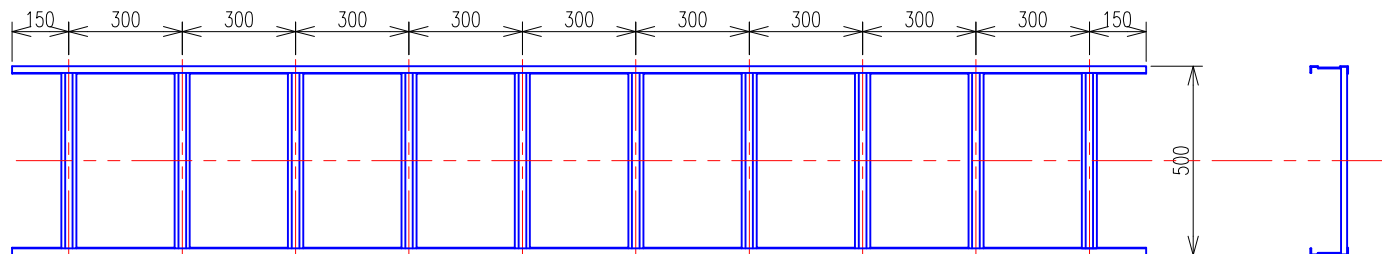
ケーブルラック (QR50) 平面図・側面図
