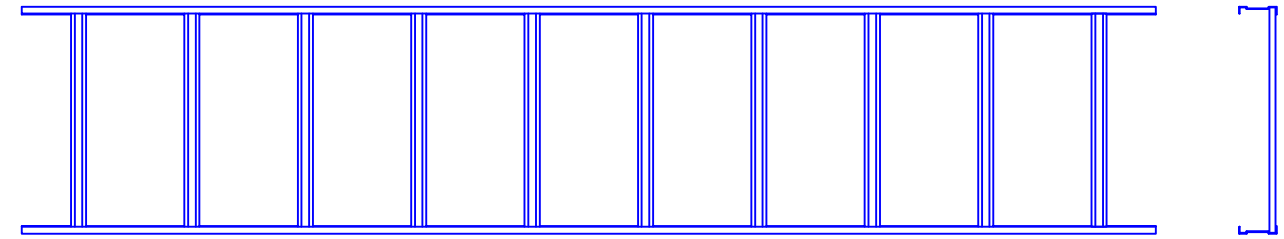
ケーブルラック (QR70) 平面図・側面図【ブロック】
