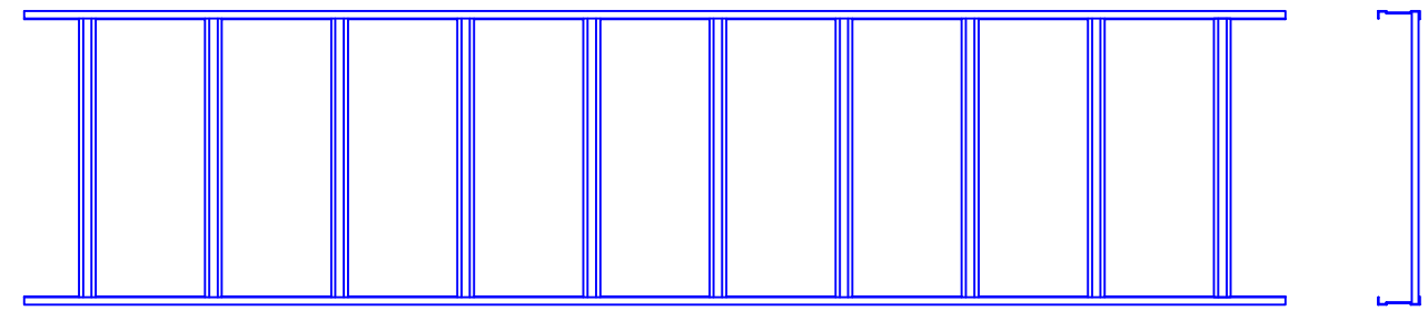
ケーブルラック (QR80) 平面図・側面図【ブロック】
