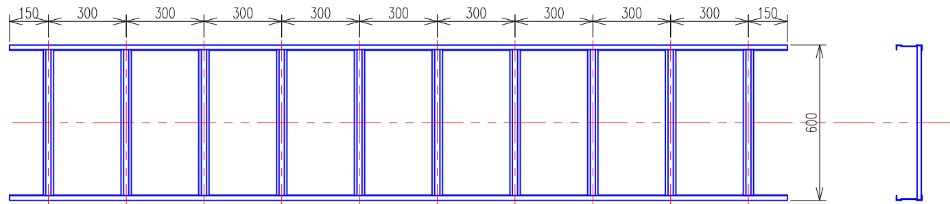
ケーブルラック (QR70) 平面図・側面図
