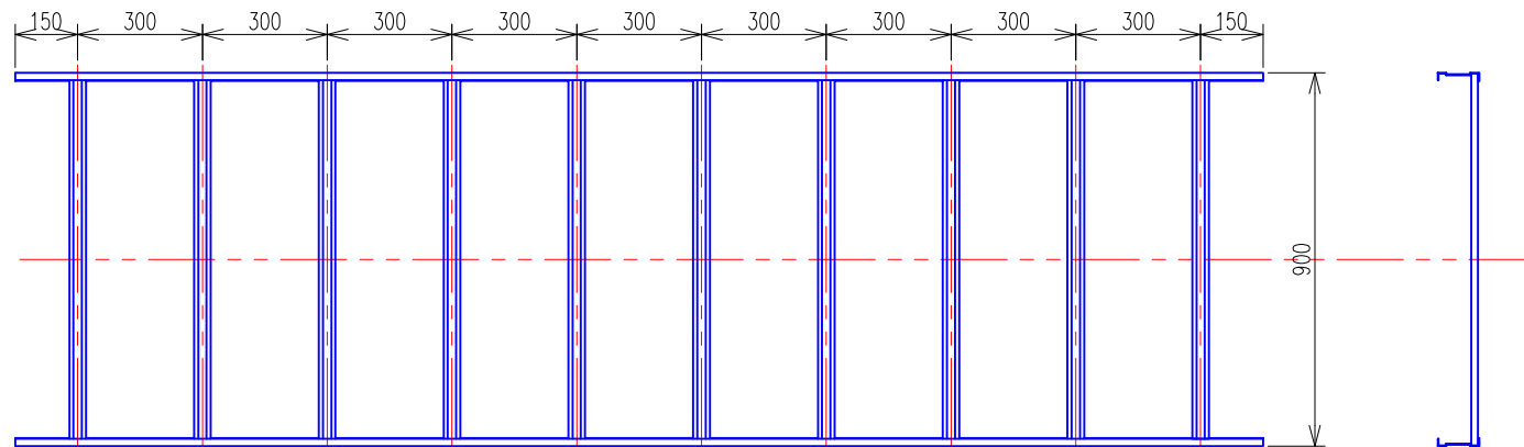
ケーブルラック (QR90) 平面図・側面図
