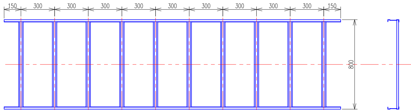
ケーブルラック (QR90) 平面図・側面図
