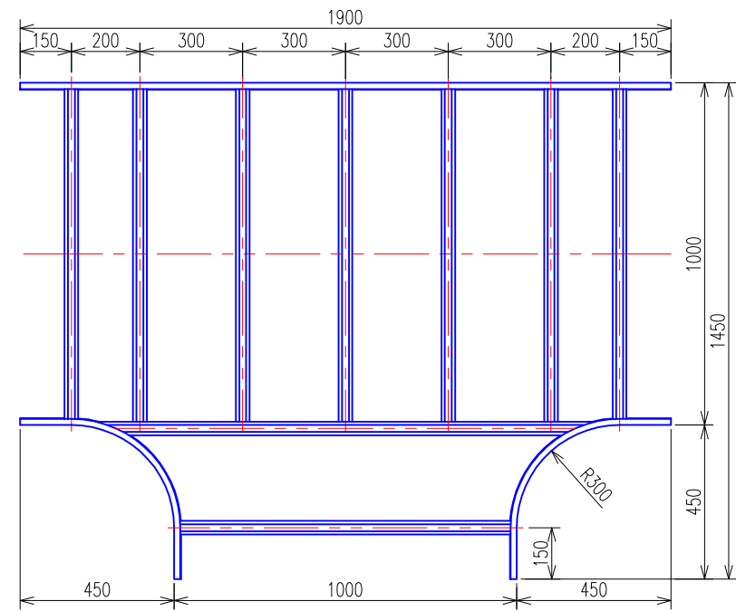
T形分岐ラック (QRT100) 平面図
