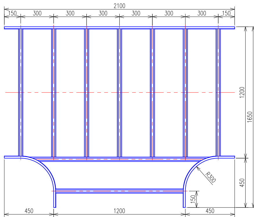
T形分岐ラック (QRT120) 平面図
