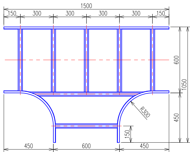
T形分岐ラック (QRT60) 平面図
