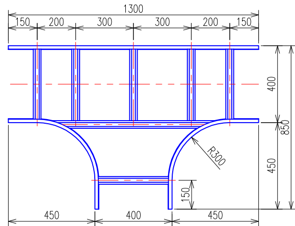
T形分岐ラック (QRT60) 平面図
