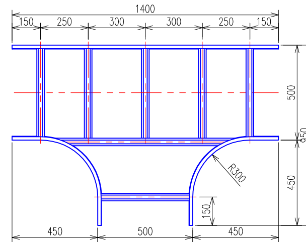
T形分岐ラック (QRT70) 平面図
