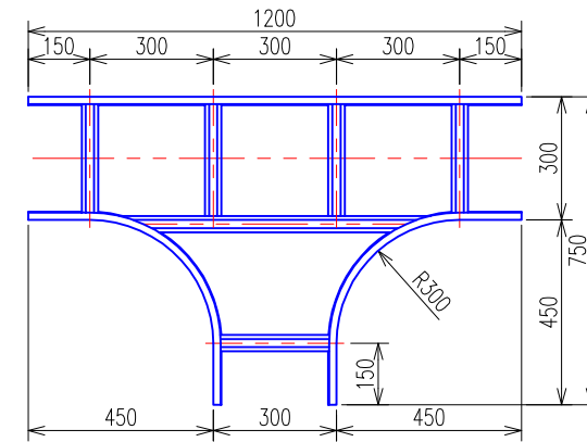
T形分岐ラック (QRT50) 平面図
