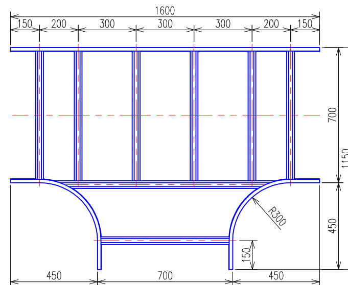
T形分岐ラック (QRT70) 平面図
