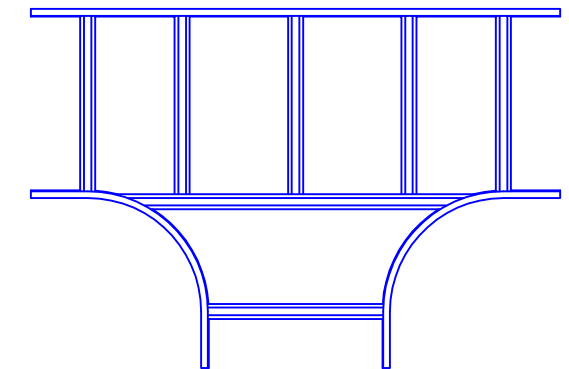
T形分岐ラック (QRT70) 平面図【ブロック】
