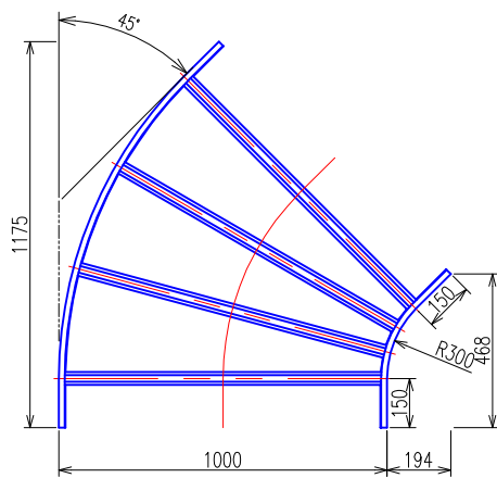
水平ベンドラック (QRA1045) 平面図
