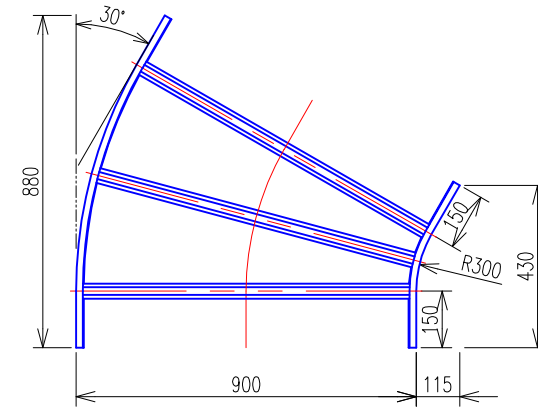
水平ベンドラック (QRA945) 平面図
