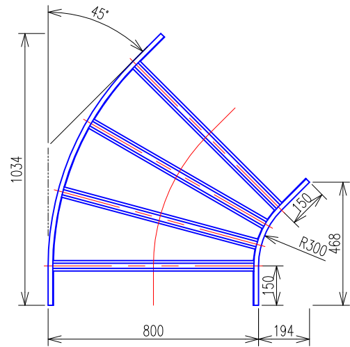
水平ベンドラック (QRA860) 平面図
