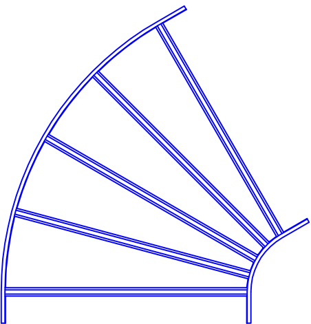
水平ベンドラック (QRA1260/1260N) 平面図【ブロック】
