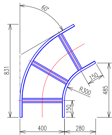
水平ベンドラック (QRA460) 平面図
