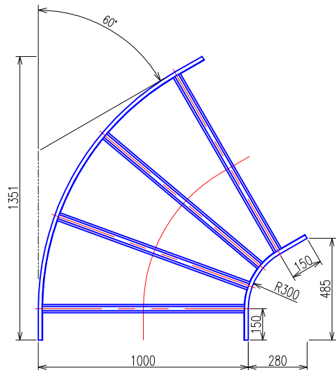
水平ベンドラック (QRA1060) 平面図
