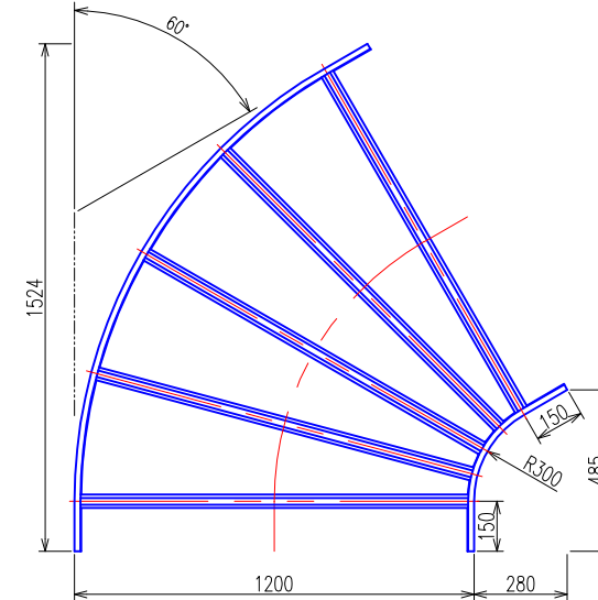
水平ベンドラック (QRA1260/1260N) 平面図
