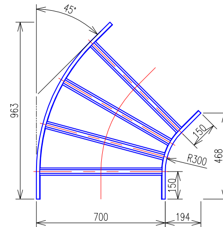
水平ベンドラック (QRA760) 平面図
