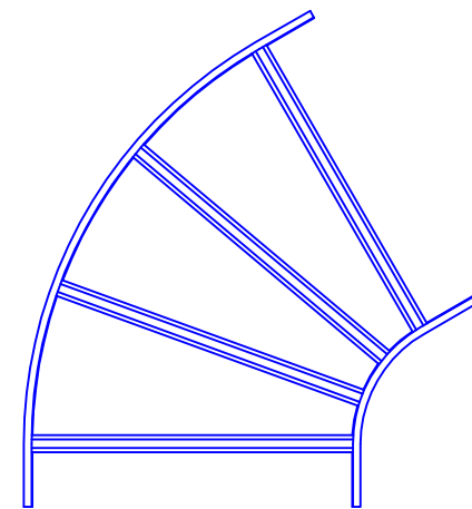
水平ベンドラック (QRA860) 平面図【ブロック】
