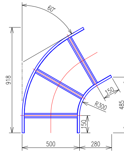
水平ベンドラック (QRA560) 平面図
