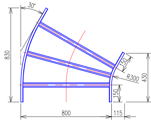
水平ベンドラック (QRA845) 平面図
