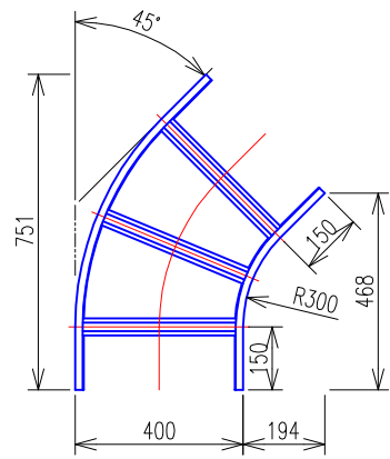
水平ベンドラック (QRA460) 平面図
