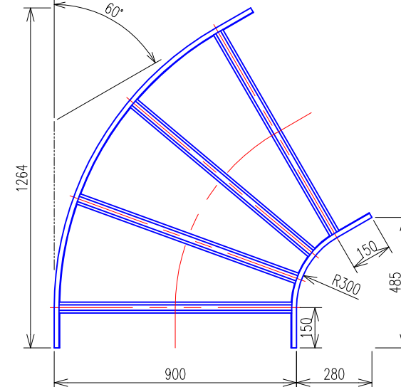
水平ベンドラック (QRA960) 平面図
