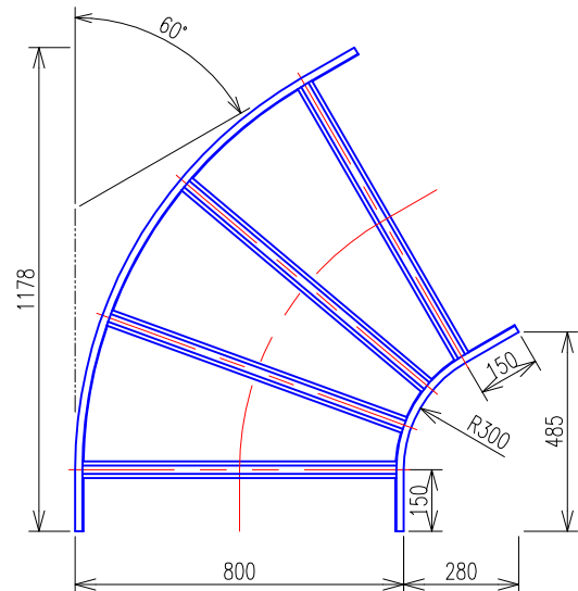
水平ベンドラック (QRA860) 平面図
