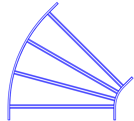
水平ベンドラック (QRA1245/1245N) 平面図【ブロック】
