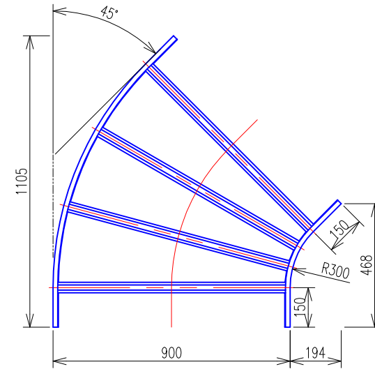
水平ベンドラック (QRA960) 平面図
