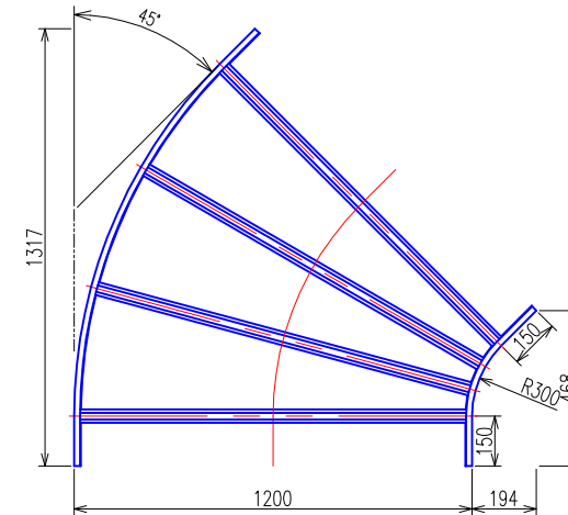
水平ベンドラック (QRA1245/1245N) 平面図
