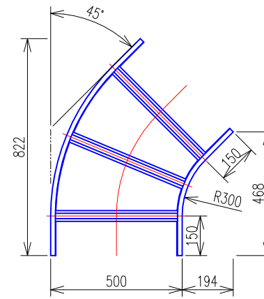
水平ベンドラック (QRA560) 平面図
