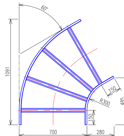
水平ベンドラック (QRA760) 平面図
