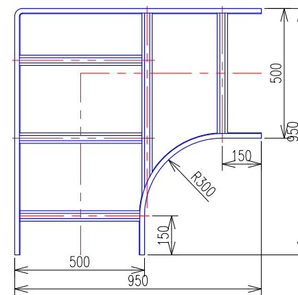
外直角L形分岐ラック (QRLA70) 平面図
