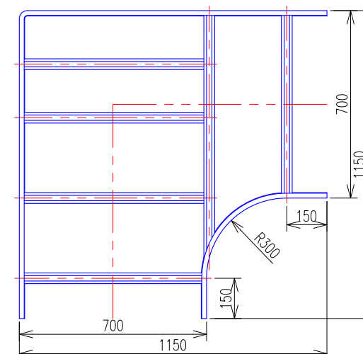
外直角L形分岐ラック (QRLA70) 平面図
