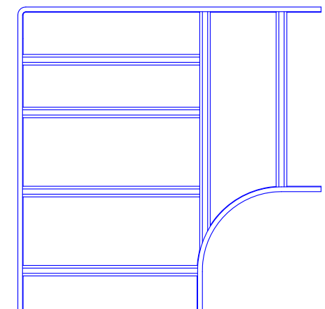
外直角L形分岐ラック (QRLA70) 平面図【ブロック】
