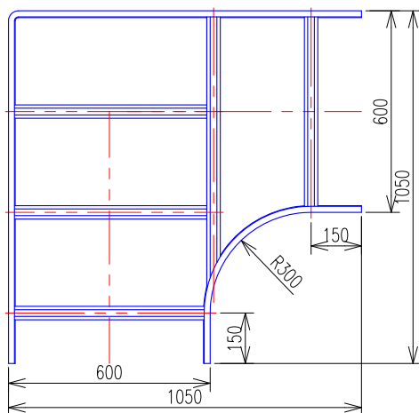
外直角L形分岐ラック (QRLA60) 平面図
